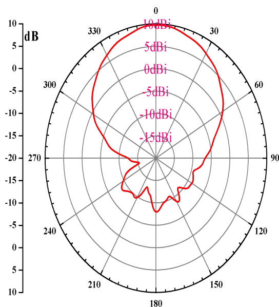
图 4 H 面二维方向图
