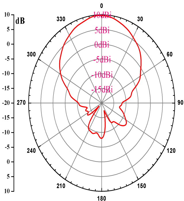
图 5 E 面二维方向图
