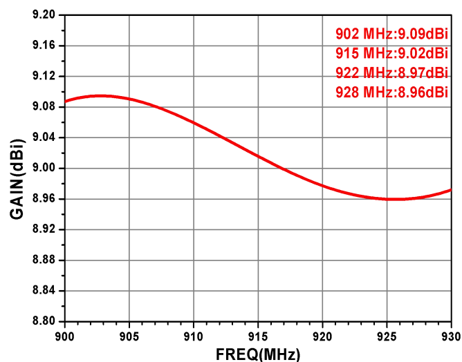
图 2 增益随频率变化曲线
