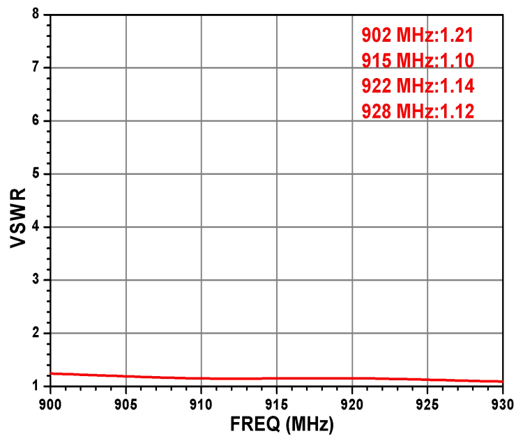
图 7 电压驻波比 VSWR 随频率变化曲线
